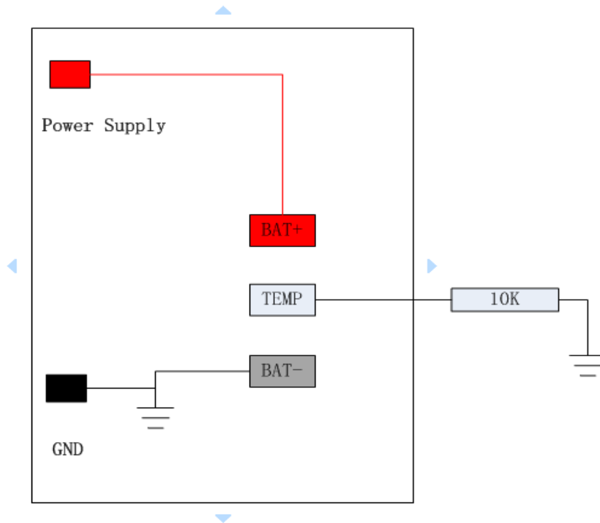
图 4.2 NTC 夹具接线方法
